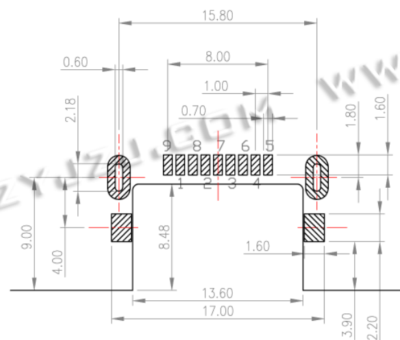
P.C.B LAYOUT
